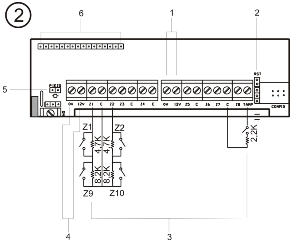
Fig. 4 Διάγραμμα Συνδέσεων IC60 compact 2
