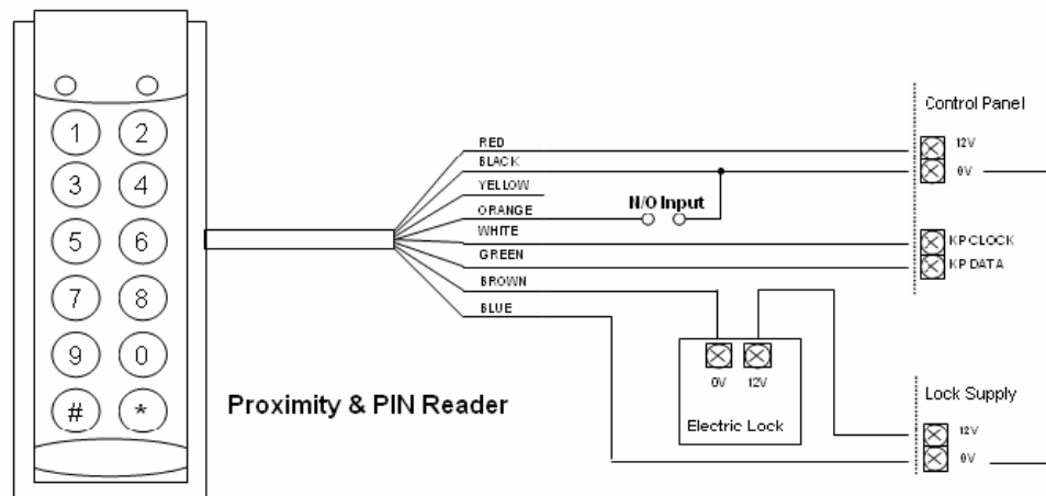
Fig. 14 Σύνδεση Επαγωγικού & Αριθμητικού Καρταναγνώστη
