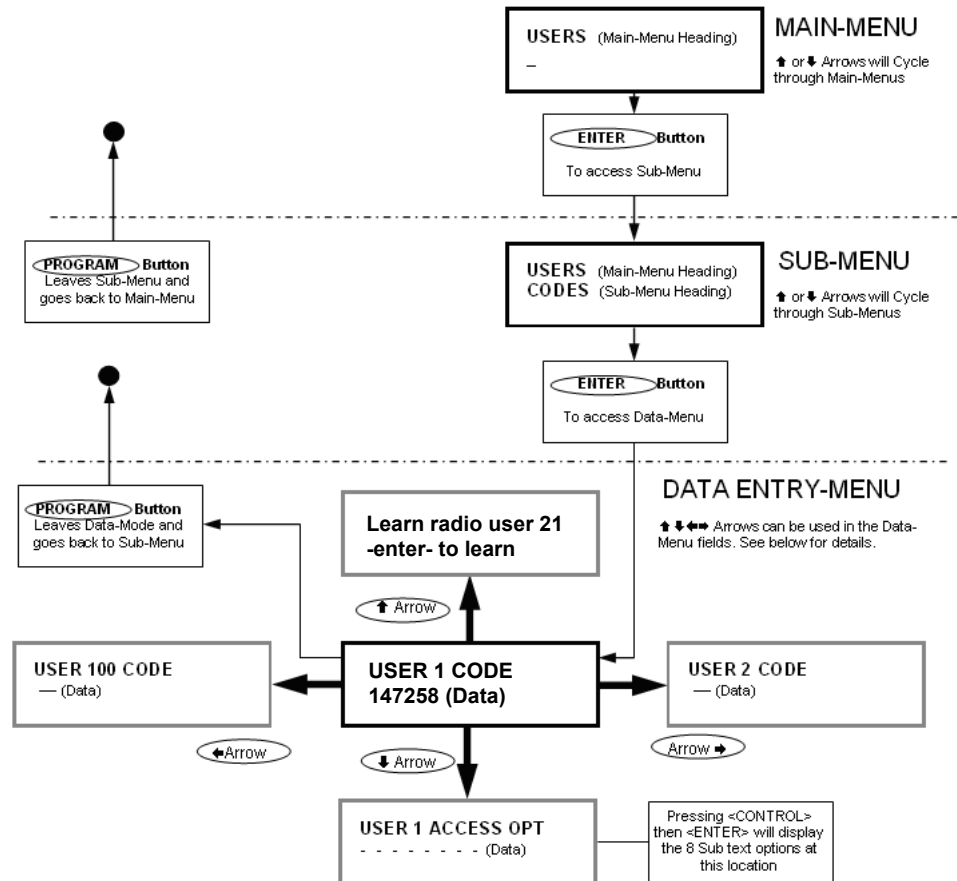
Fig. 19 Διάγραμμα ροής με βήματα σε Καταλόγους (menu) χρησιμοποιώντας τα πλήκτρα: Βέλος, Enter και Program
